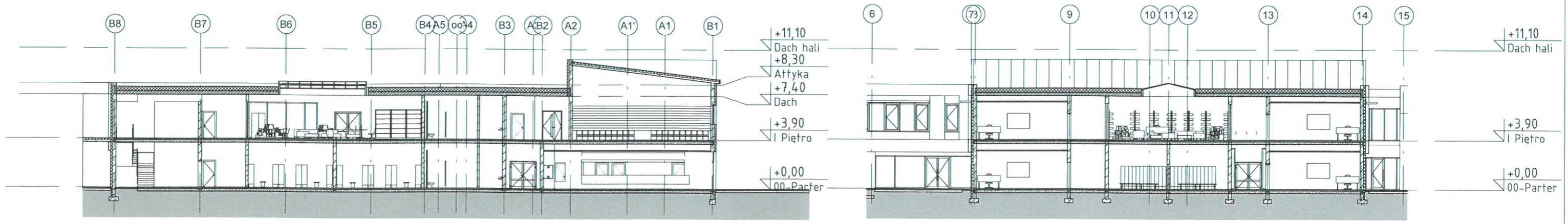
2 B1 1:300
